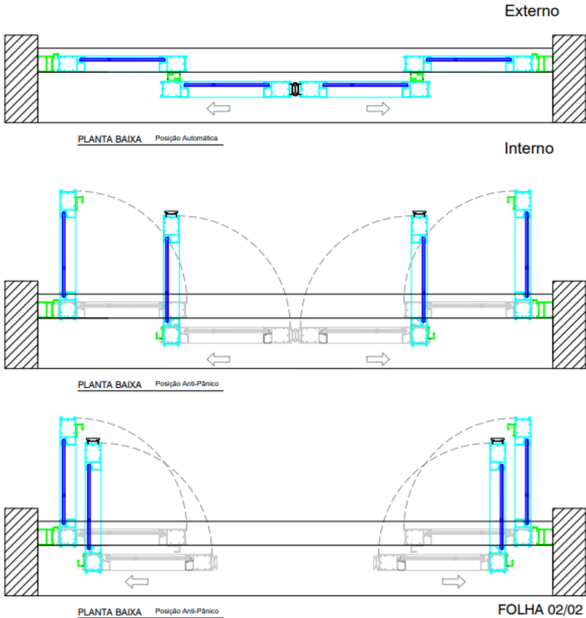
Figura 1. SISTEMA ANTIPÂNICO PARA PORTA SOCIAL CÂMARA MUNICIPAL DE PAULÍNIA.
